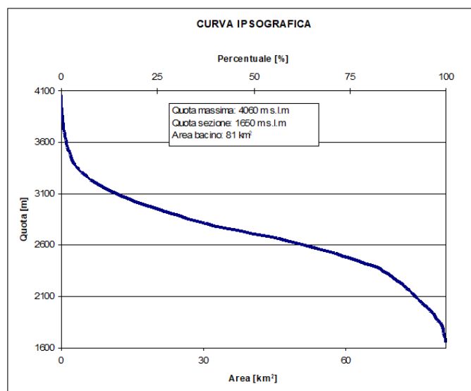
Curva ipsografica del bacino sotteso dalla sezione idrometrica di Valsavarenche - Eaux-Rousses.
